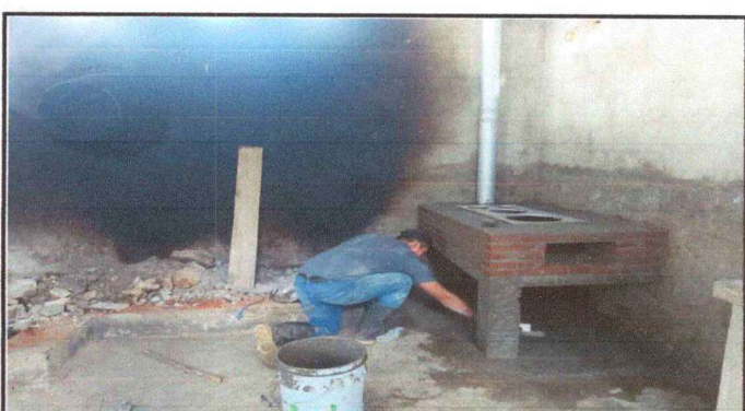
Foto 4: Proceso de elaboración de estufa completa con plancha de metal y chimenea.
